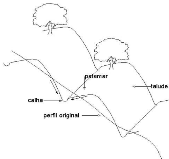
Figura 53: Corte esquemático de terreno e construção de patamares.
